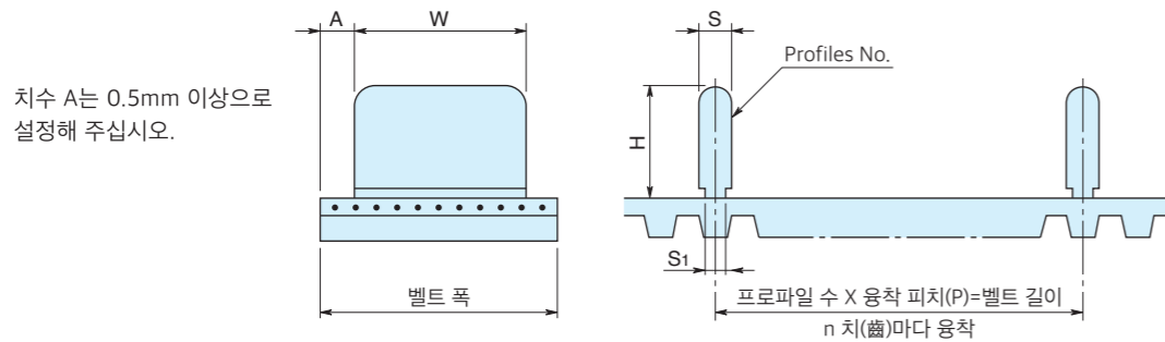
프로파일의 용착 전 공차
