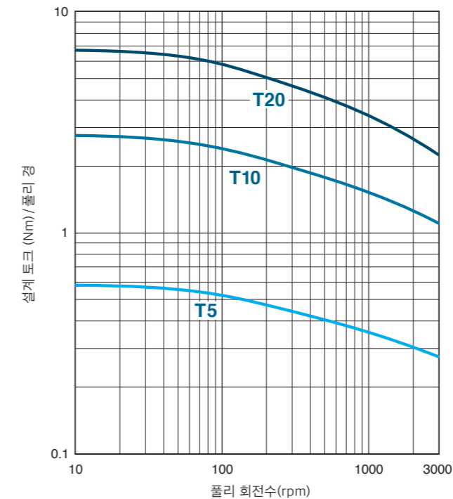
선정 도표 2-3: 미터(meters)에 따른 벨트
