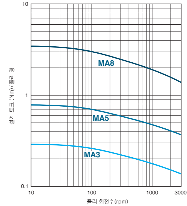
선정 도표 2-1: MA 벨트
